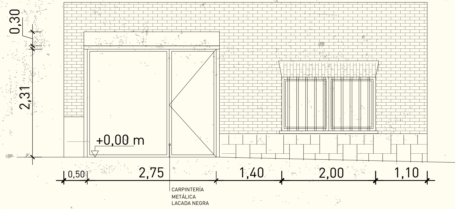
ALZADO 1
